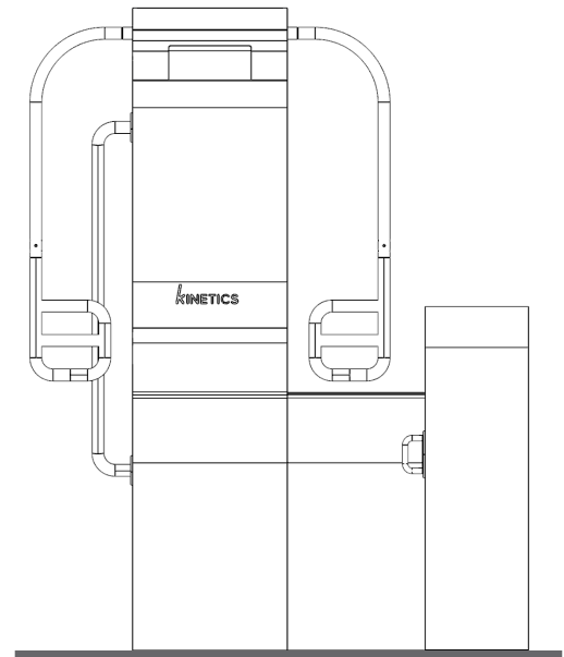
Right Elevation
